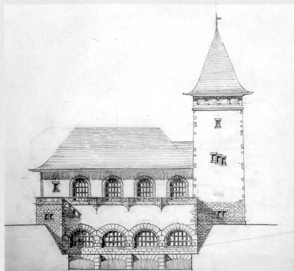
Avant-projet pour l'usine de l'Oelberg, version du bureau Broillet & Wulffleff, novembre 1907 (AEF)
