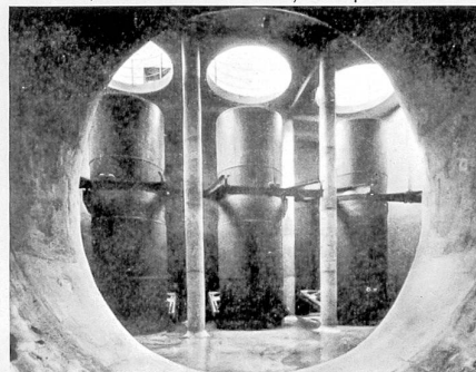
La chambre de mise en charge, haute de 9,40 m, vue du tunnel, avec ses trois vannes cylindriques en métal
