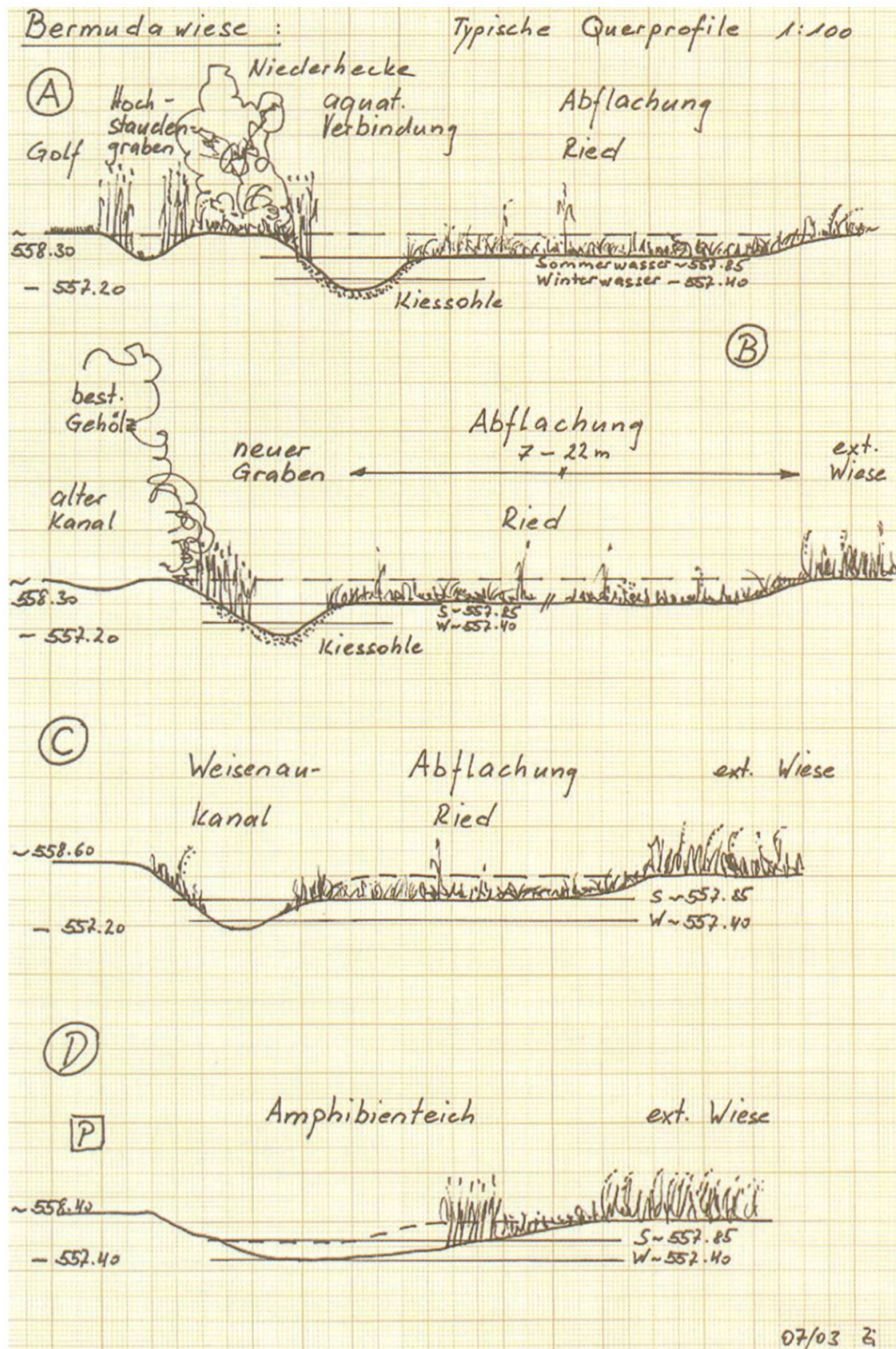
Abb.15: Typische Querprofile im Rahmen des Renaturierungsprojektes Bermudawiese.
