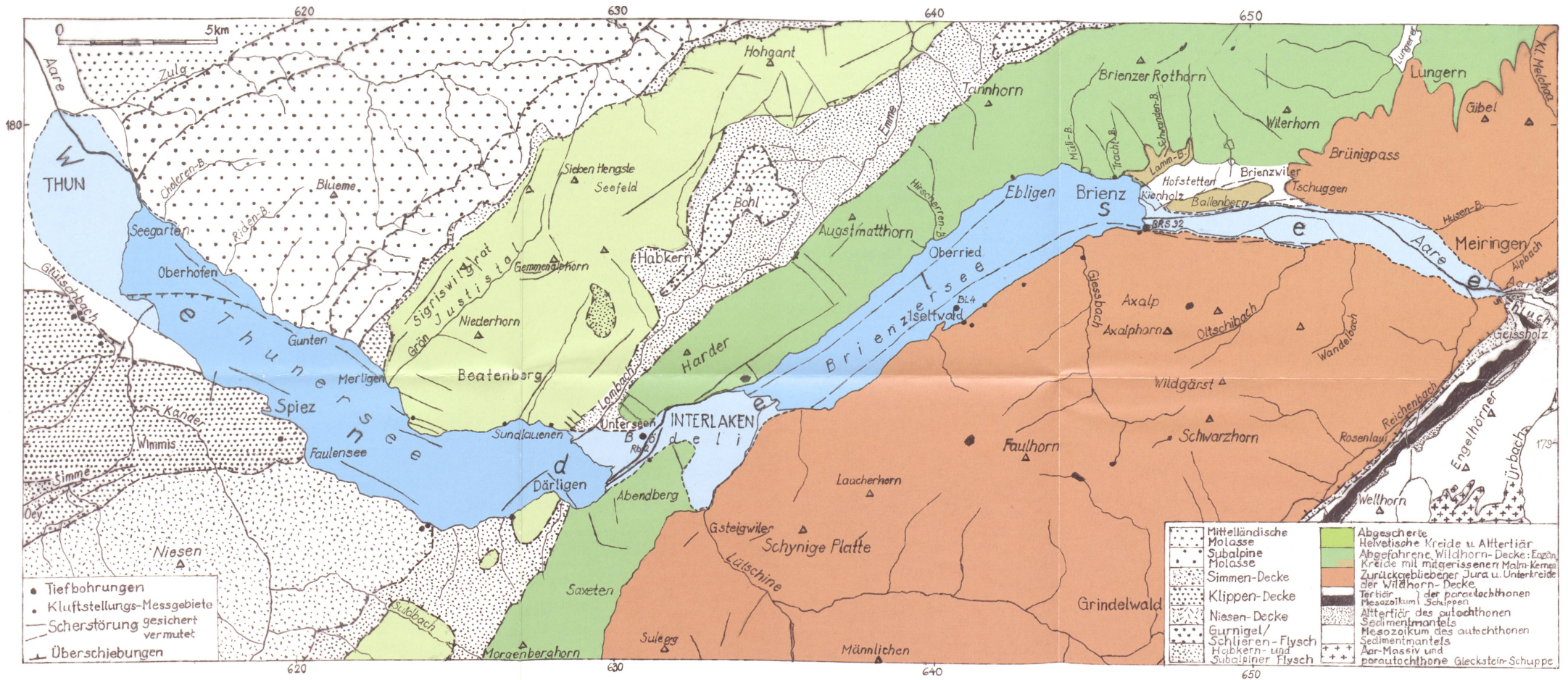
Tafel 1 Tektonische Übersichtsskizze des Gebietes von Brienz- und Thunersee, Überreste des einstigen Wendelsees, • Messstellen der Klüftstellungen und den Tiefbohrungen
