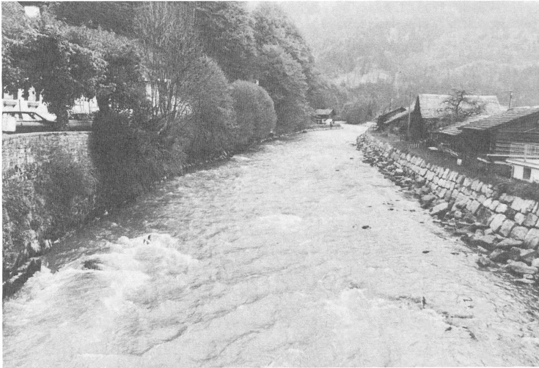
Die Lütschine bei Gsteig. Blick flussaufwärts. Links bildet der Fuss des Aenderbergs ein natürliches Ufer, rechts wurde ein starker Damm gebaut, um die angrenzenden Häuser und das Bödeli vor Überschwemmungen zu schützen.
