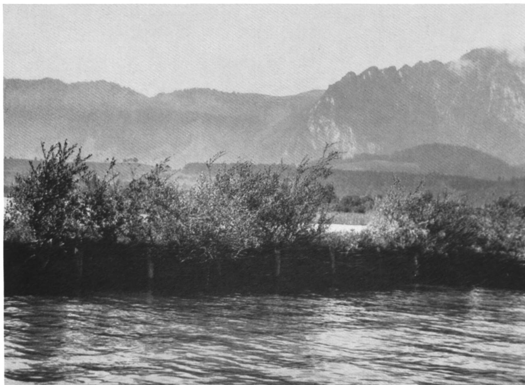
Etterwerk als Ufersicherung ist noch besser
