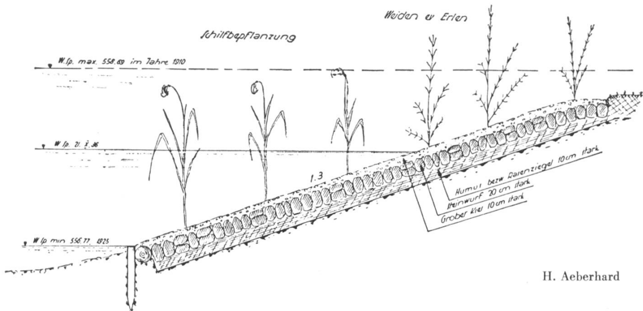
Vorbildliche Ufersicherung
