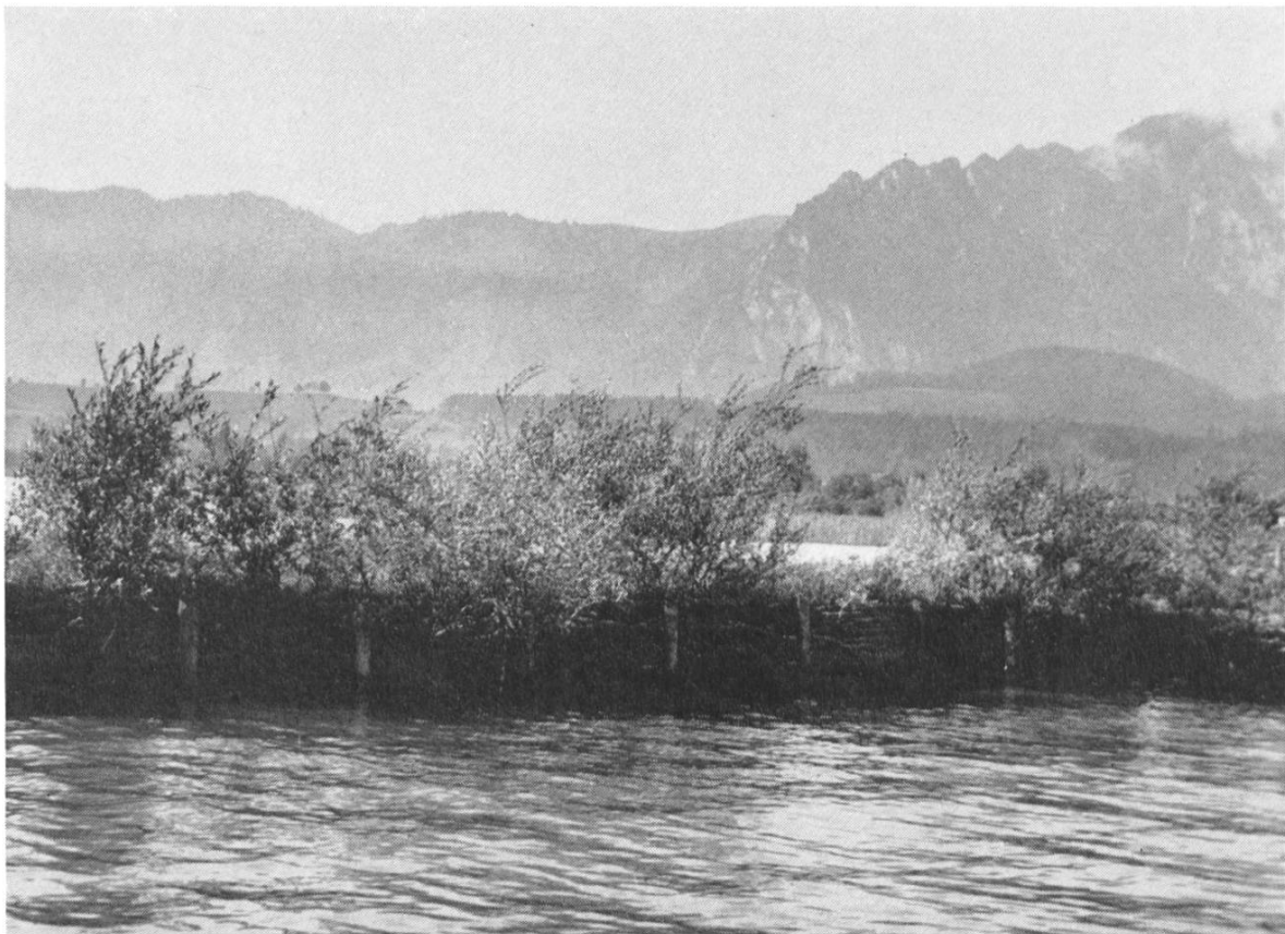
Etterwerk als Ufersicherung ist noch besser
