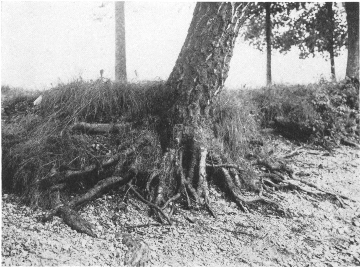
Am Strandweg Bönigen U. Brunner Vom Wellenschlag unterspülte Baumwurzeln. Hier haben wir Ufersicherungen gebaut
