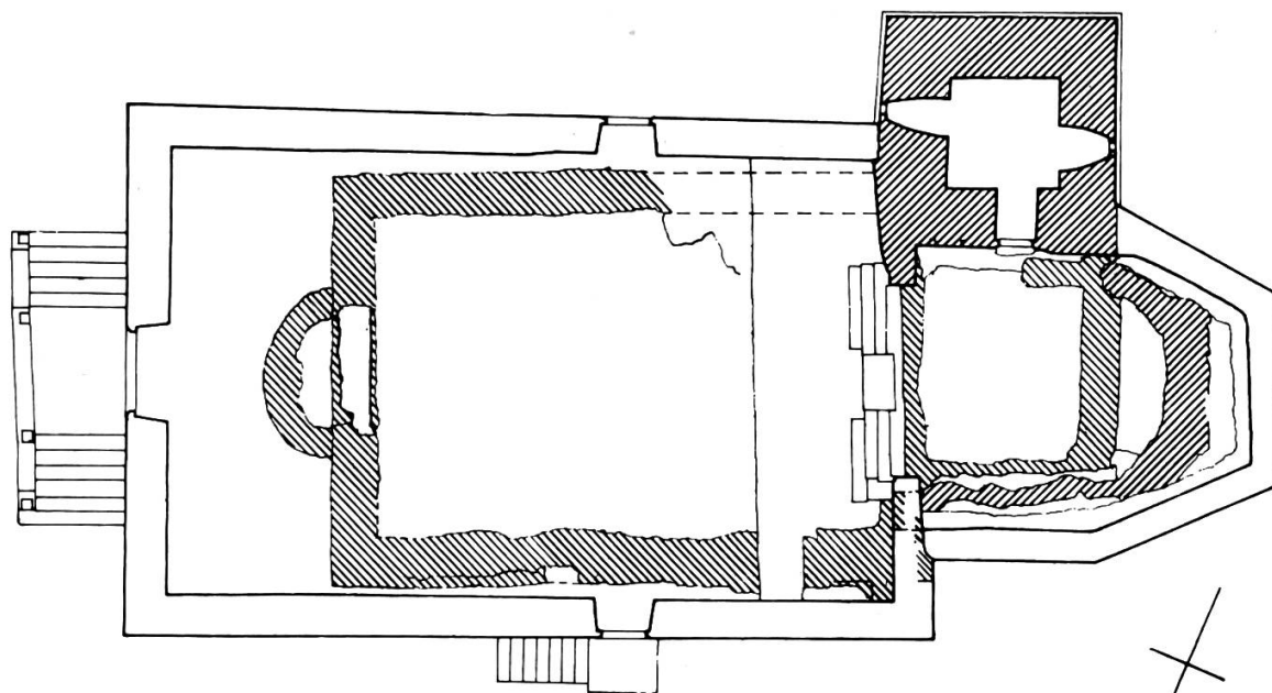
BOSWIL EHEM. PFARRKIRCHE ST. PANKRAZ ARCHÄOL. GRUNDRISS
