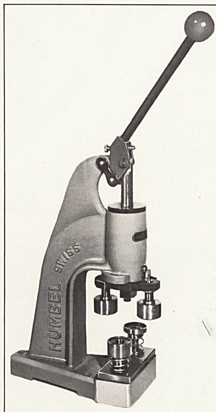
Schwenkpresse mit Handbetätigung
