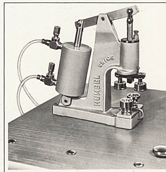
Schwenkpresse mit Pressluft-Antrieb
