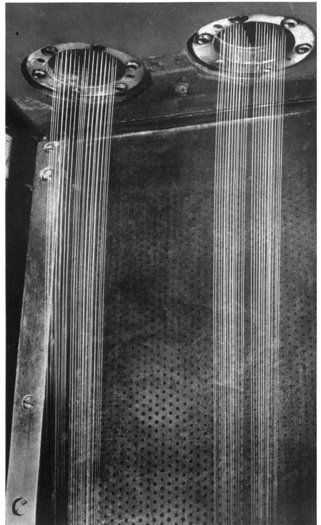
El nylon fundido sale de las hileras y se solidifica inmediatamente al enfriarse
