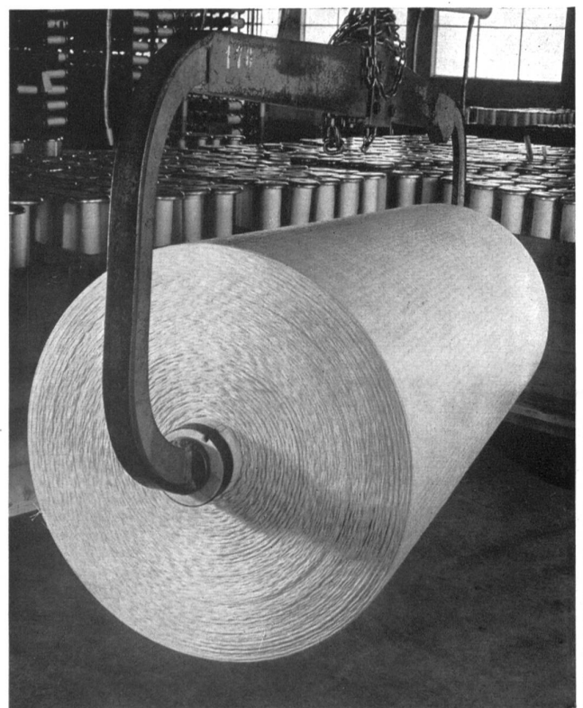
Rollo de tela para neumáticos, de «Viscor», hilo de viscosa de rayón de elevada tenacidad
