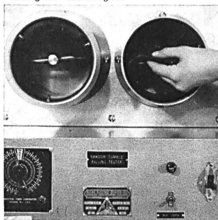
Pillingprüfung
