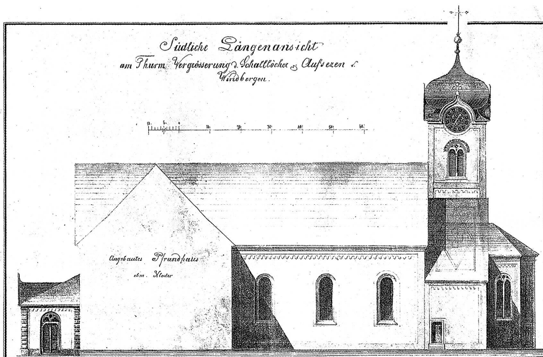
Pfarrkirche Alt St. Johann. Südaufsicht der neuen Pfarrkirche, erbaut 1869/70 von Carl Reichlin. – Nach Originalplan im Kirchgemeindearchiv.
