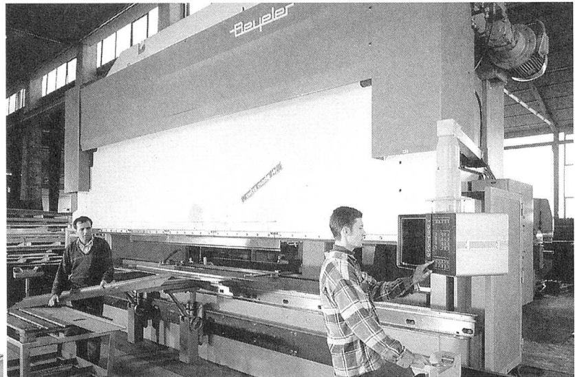
Abkantpresse Beyeler, 600 t x 7200 mm
