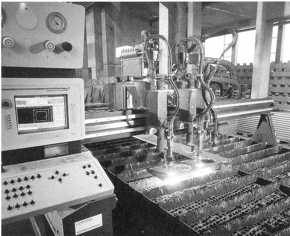
CO 2 -Laser-Schneidanlage
