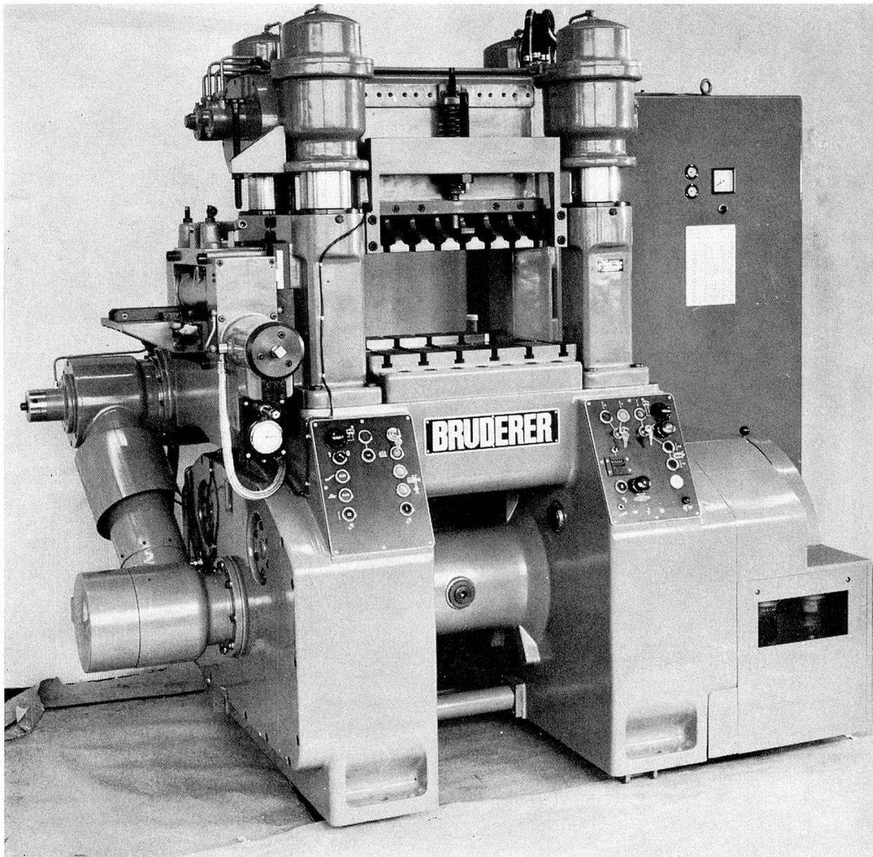
Typ BSTA 60
