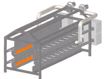
Abb. 4: Kombinierte Luft-Infrarottrocknung
