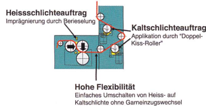
Abb. 3: Prinzip des Heiss- und Kaltschlichteauftrags im Beschlichtungszentrum
