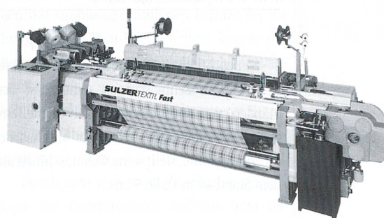
Abb. 3: Greiferwebmaschine FAST (vormals Nuovo Pignone)
