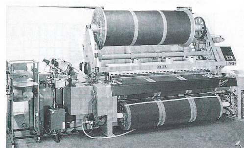
Abb. 10: Picanol-Günne Frottierwebmaschine (Luftdüse)
