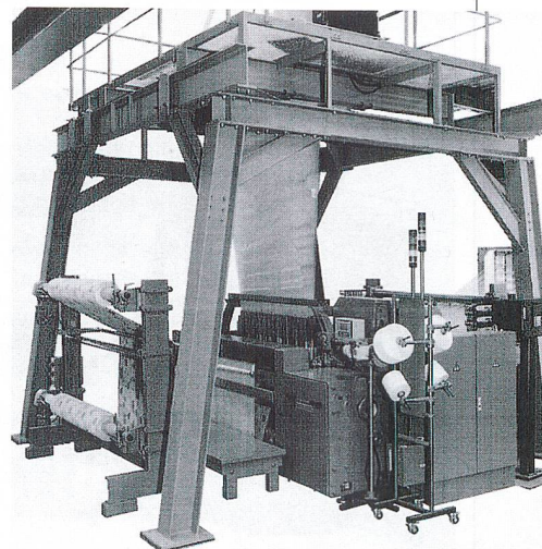
Abb. 11: Picanol-Günne Doppelflo-Greiferwebmaschine
