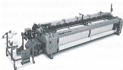
Abb. 5: Projektilwebmaschine
