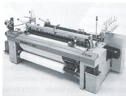
Abb. 4: L5200 Luftdüsenwebmaschine von Sulzer Textil
