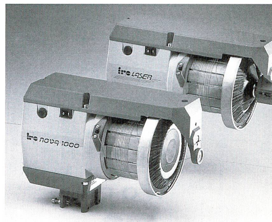
Schussfadenspeicher Laser/Nova Foto: IRO
