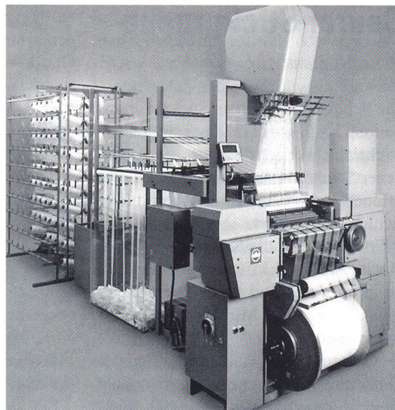
Jacquard-Kettenwirkmaschine Raschelina RD3J (MT2)
