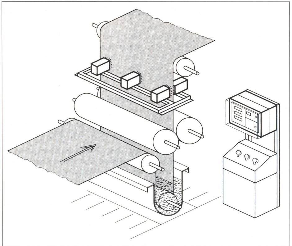
Flottenauftragsmessung und -regelung am Färbefoulard mit AF 310 Foto: Pleva
