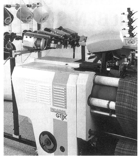
Bild 4: Schussfadenspeicher mit Quick Step Einrichtung
