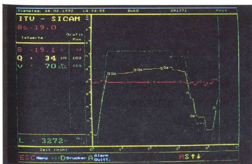
TELECOLL-Beschlichtungssteuerung
