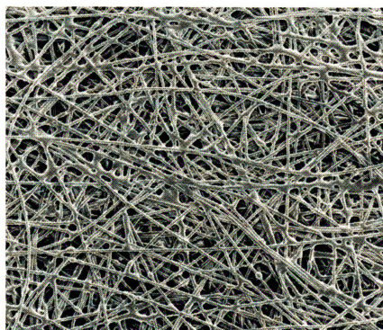
Die Endlos-Polyesterfasern der Lutradur-Teppichträger von Freudenberg haben eine sehr gleichmässige Struktur. Teppichen verleihen sie Dimensionsstabilität und eine homogene Oberfläche.
