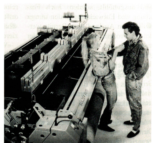
Zwei Drittel aller Denimgewebe werden heute weltweit auf Sulzer Rüti-Projektwebmaschinen hergestellt. Bild: Sulzer Rüti, Rüti
