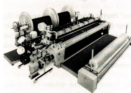
Sulzer Rüti-Projektilwebmaschine mit Schussmischer, zweibahnig belegt mit einem Denim, ausgerüstet mit Exzentermaschine, Motor-Kettablass Grob, automatische Schuss-Suchvorrichtung, automatische Fach-Hebevorrichtung, Webkettenspanner, Schusspeicher TMT, separater Kettbaumanordnung und Dockenwickler Grob.
