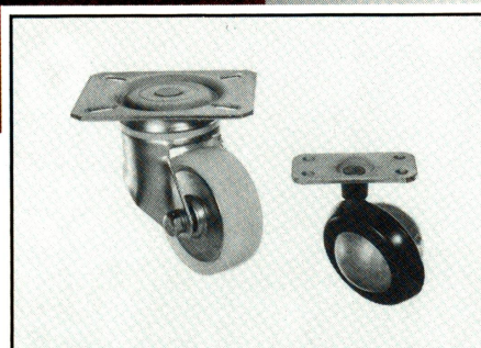
Besonders robuste Gabelkrolle (links) Verbesserte Kugellenkrolle (rechts)
