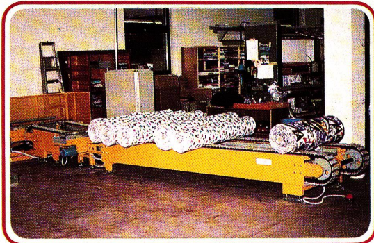
Detail der Transportsanlage der Textildruck Schellenberg - CH - Fehrltorf.
