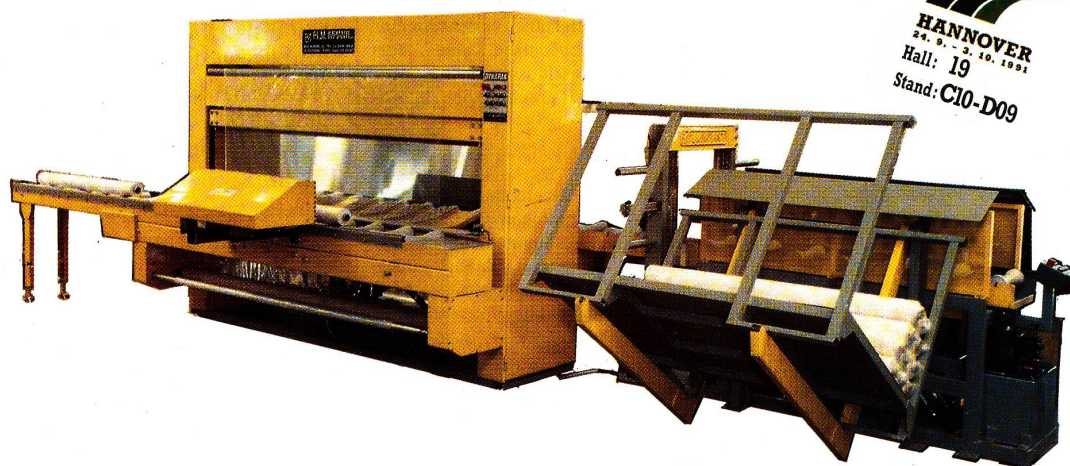
Verpackungsstraße Typ DYNAPAK 500 AL
