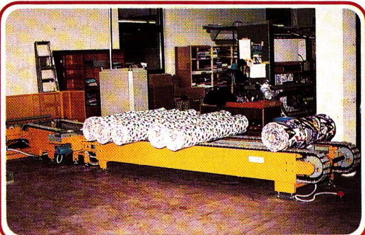
Detail der Transportsanlage der Textildruck Schellenberg - CH - Fehraltorf.
