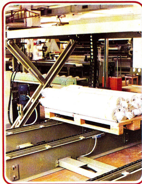
Palettiervorrichtung Typ PTN 48
