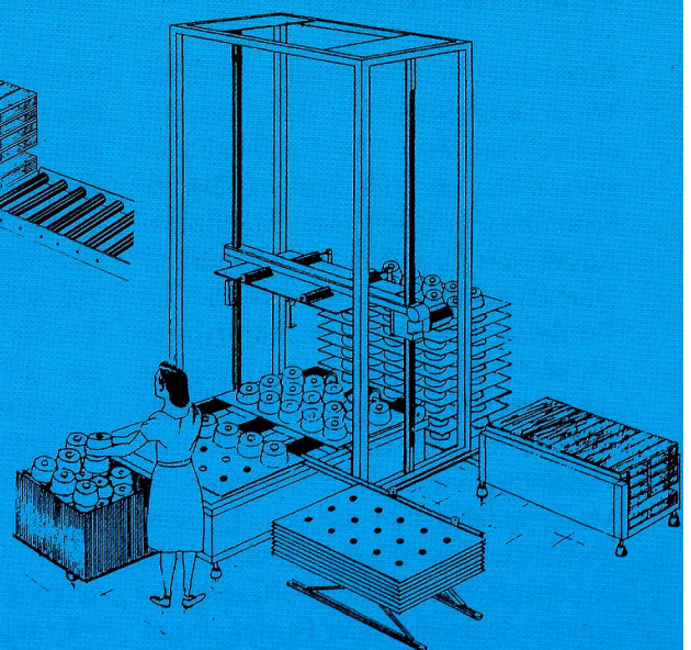
Verpackung auf Paletten Halbautomatischer Palettierer Mod. PH3
