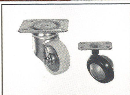
Besonders robuste Gabelnrolle (links) Verbesserte Kugellenrolle (rechts)
