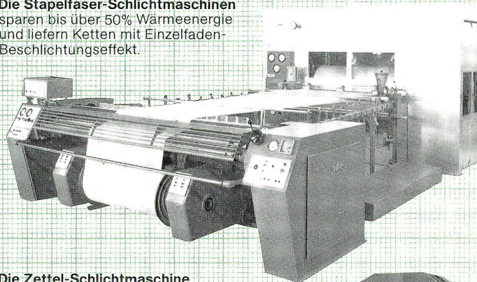
● Die Zettel-Schlichtmaschine beschlichtet prozeßsicher mit 400 m/min Filamentgarne mit programmierten Daten.
