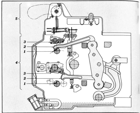
Die klare Gliederung der Schaftmaschine in eine Antriebsgruppe 4 und eine Steuergruppe 5 ist das Merkmal dieses funktionsorientierten, bedienungsfreundlichen und übersichtlichen Konzeptes.
