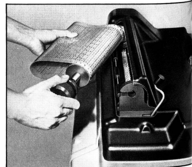
Die kompakte, für hohe Arbeitsgeschwindigkeiten ausgelegte Steuergruppe 5 zeichnet sich durch den kontinuierlichen Vorschub der Musterkanten und den schwenkbaren Kartenzylinder aus.
