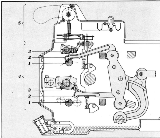
Die klare Gliederung der Schaftmaschine in eine Antriebsgruppe 4 und eine Steuergruppe 5 ist das Merkmal dieses funktionsorientierten, bedienungsfreundlichen und übersichtlichen Konzeptes.
