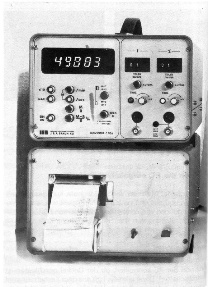
Digitales Messgerät für Drehzahl, Geschwindigkeit, Verhältnis, prozentuale Differenz zum beweglichen Einsatz, dazu Messwertdrucker
