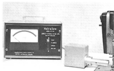
HATRASEW Stichschaden-Prüfgerät
