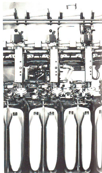
AUTOCONER GKT mit Splicerautomatik. Das Y-Magazin nimmt Garne mit einer Y-Koppe bis 600 mm Länge auf.
