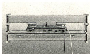
Heizpresse PP-1200 für minutenschnelles Endverbinden. Nutzbreite: 1200 mm.
