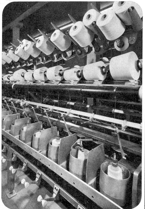
Doppeldraht-Zwirnmaschine
