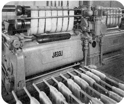
Garmmercerisiermaschine
