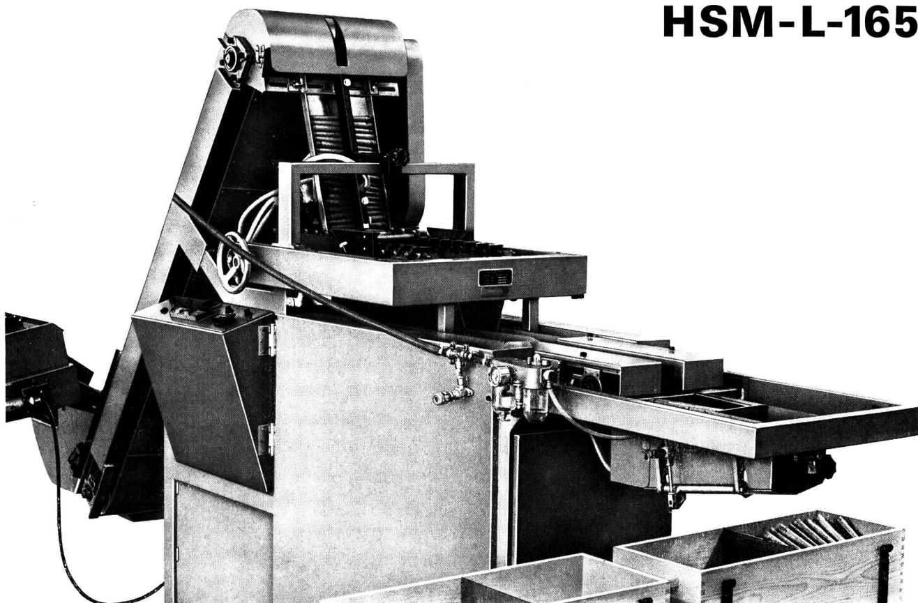
Zähl-, Sortier- und Ablegezone des neuen Modells HSM-L-165
