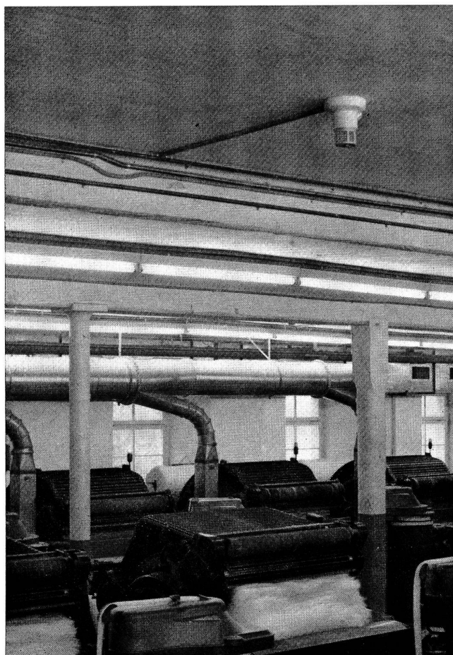
Die praktische Anwendung: der Melder auf unserem Bild sorgt dafür, dass, wenn in seinem Ueberwachungsbereich ein Feuer entsteht, dies sofort an die Löschequipen gemeldet wird. So ist es möglich, dass das Feuer bekämpft werden kann, noch bevor der Sachschaden grössere Ausmasse annehmen kann. (Foto Cerberus AG)
