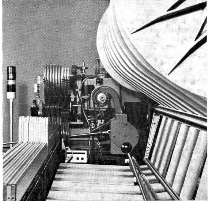
Diese Seitenansicht zeigt den einfachen Lauf der Polkette sowie das zentrale Frottieraggregat
