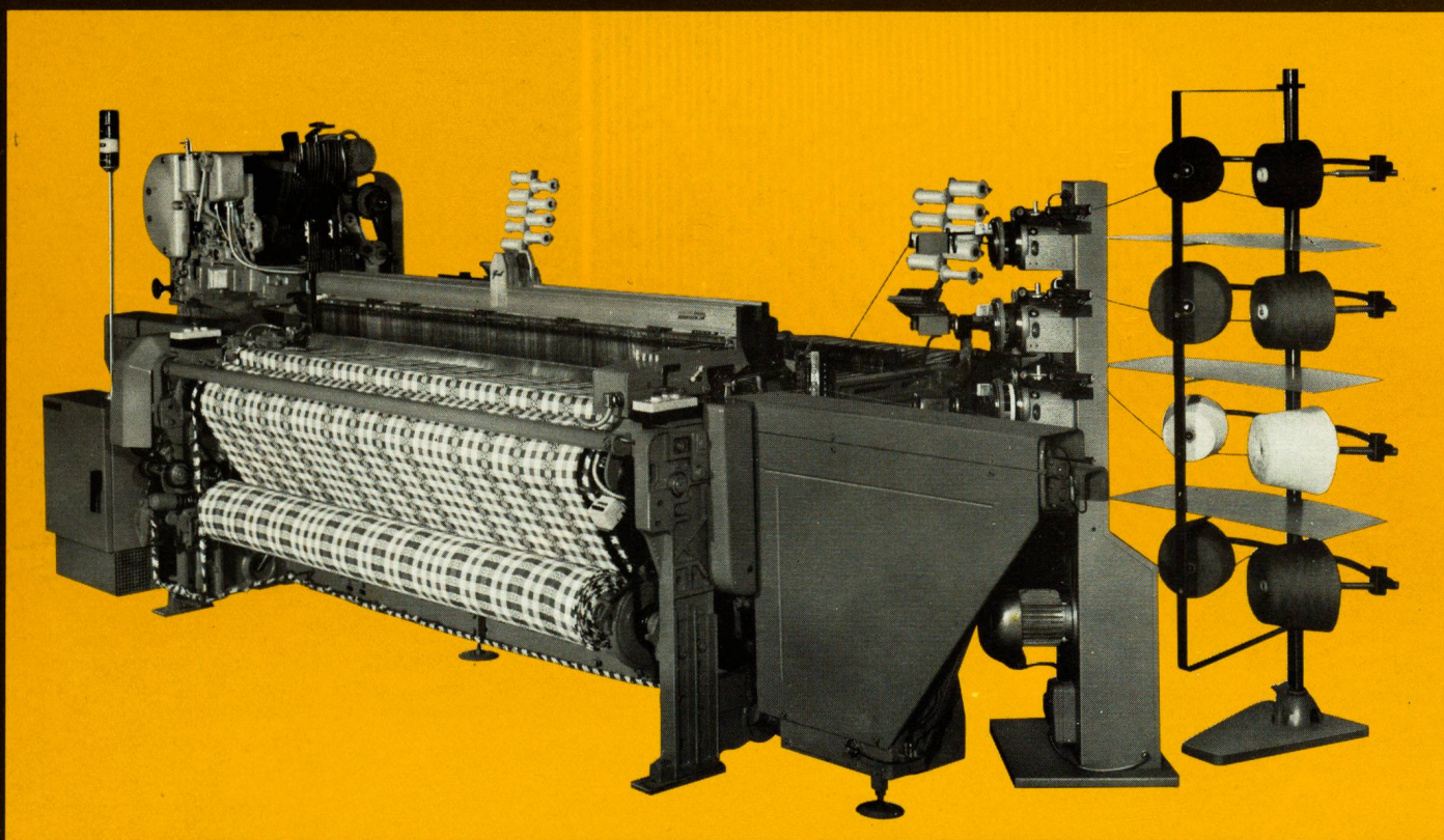
Schützenlose Mehrfarben-Webmaschine Typ VERSAMAT
