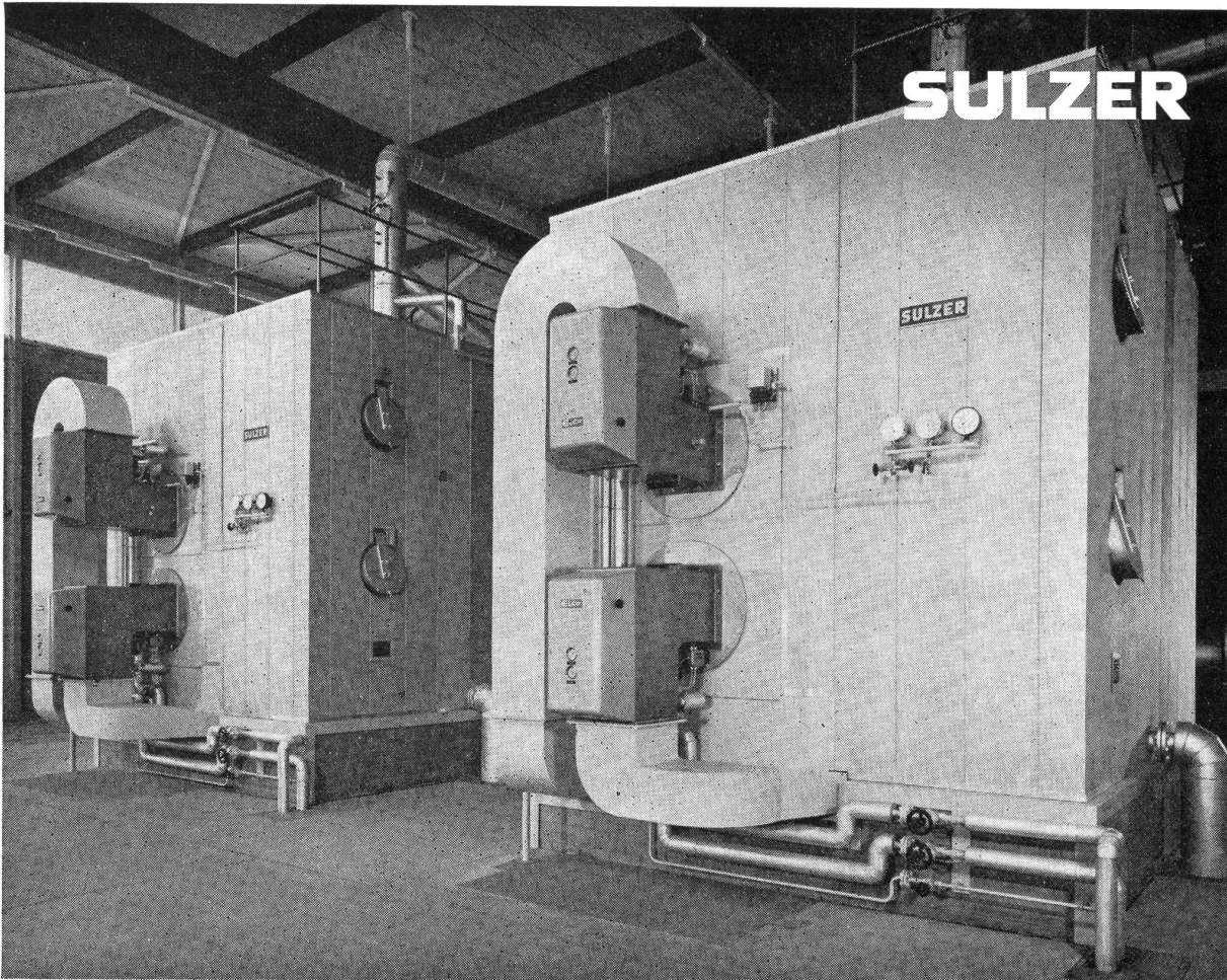
Heißwasser-Röhrenkessel in einem Industriebetrieb mit einer Leistung von je 8 Mio kcal/h, Betriebsdruck 25 atü.
