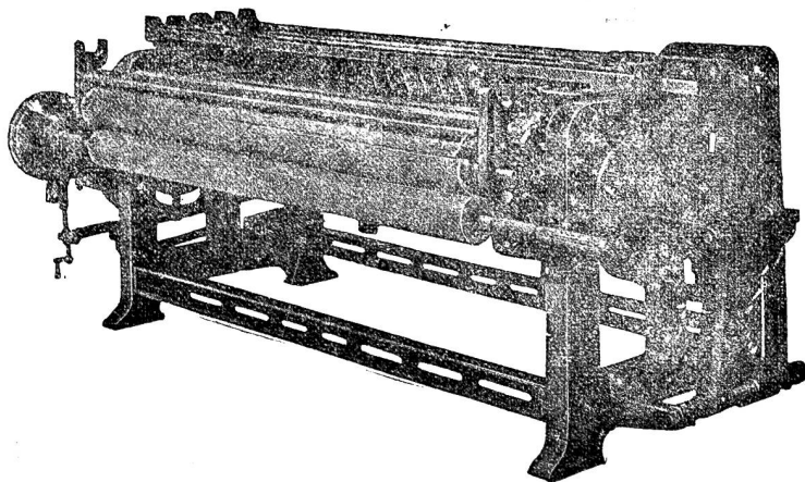
Querschnittsmaschine gegen die Rille laufend mit Messerschleifen System Simonin
