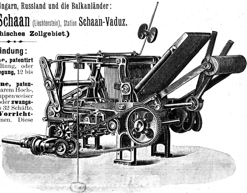
Offenfach-Schaftmaschine, doppelhebend, mit zwangsläufiger Cylinderbewegung. Gros-de-tour-Vorrichtung und Hakenauskehrung.
