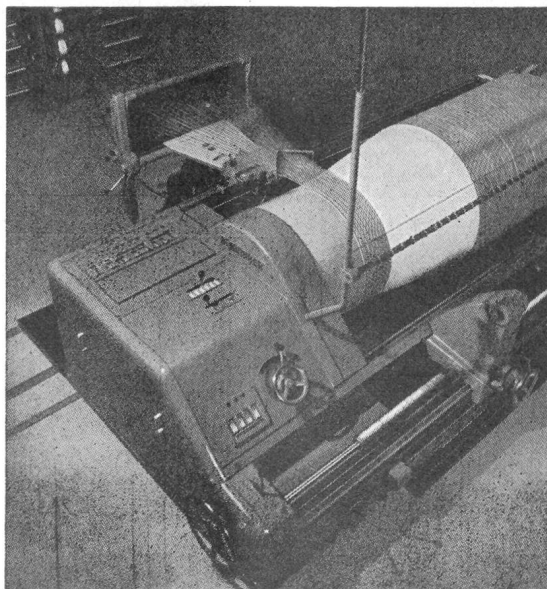
Konusschärmaschine, Modell ZA
