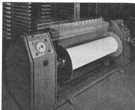
Konusschärmaschine, Modell ZA
