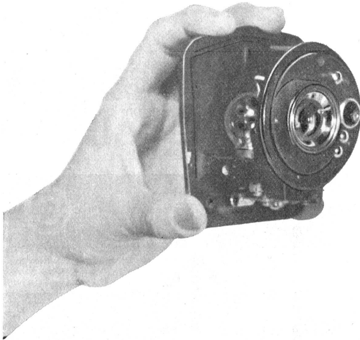
Auswechselbare Verstärker- einheit im Abtastkopf
