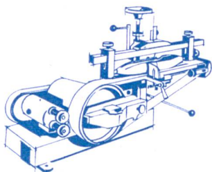
Webschützen-Abrichtmaschinen System Spaleck, auch mit Staubabsaugvorrichtung
