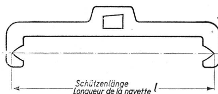
Kontroll-Lehre
