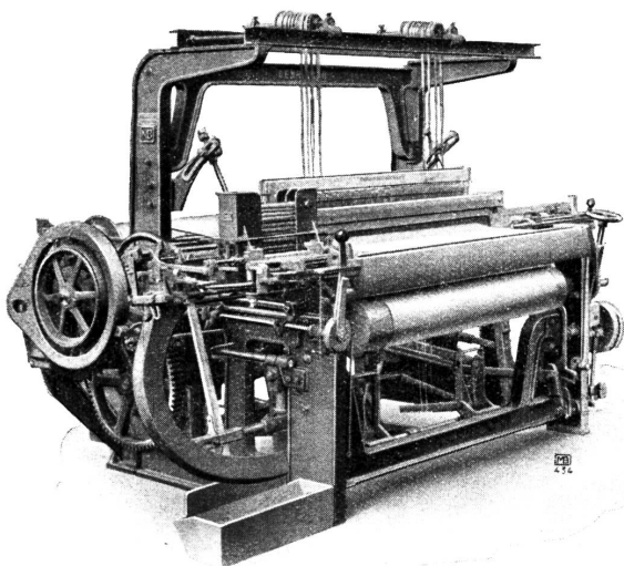
Benninger-Schützenwechsel-Seidenautomatstuhl für glatte- und Crêpe-Artikel
