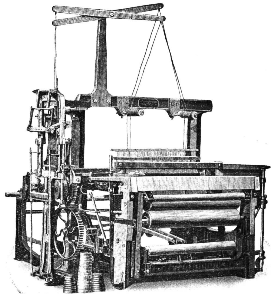
Benninger-Seidenwebstuhl Modell 1869—1880
