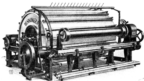
Benninger-Hochleistungs-Zettelmaschine
