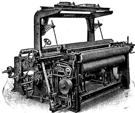
Spezial-Seidenwebstuhl für Crêpe de Chine mit Regulator für direkte Warenaufwicklung.
