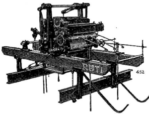
Hoch-, Tief- und Schrägfach-Jacquardmaschine, Modell JFS, mit Stangenantrieb
