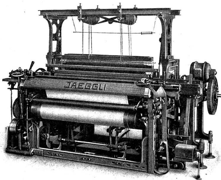
Hochleistungs-Schnellläufer-Seiden-Grèpestuhl „Universal“ 126 cm, mit elektrischem Zahnrad-Einzelantrieb
