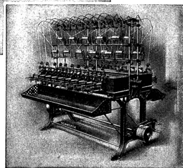
Kreuzschuß-Spulinmaschine Typ BUA. „Klein-Rapid“
