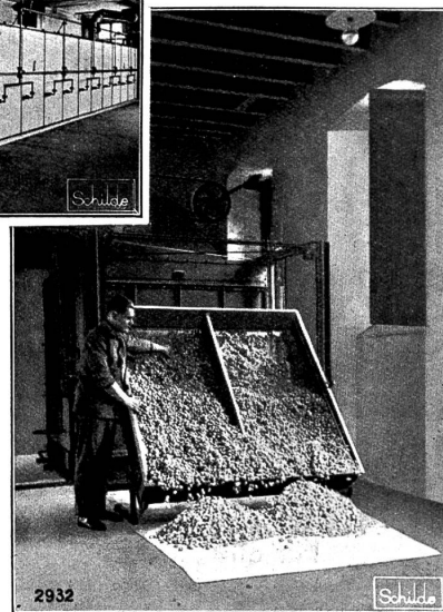
Schilde Hordentrockner Simplior zum Trocknen und Abtöten von Kokons
