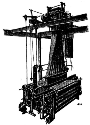
6-schütziger Spezialstuhl für Möbel- und Korsettsstoffe, Modell DWSC, kombiniert mit RÜTI-Jacquardmaschine
