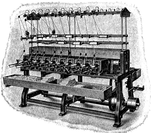
Kreuzschußspulmaschine Mod. CK 155
