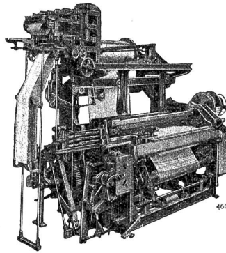
4-schütziger automatischer Webstuhl für Frotterwaren, Modell BAWF/4, kombiniert mit Rütli-Schaffmaschine
