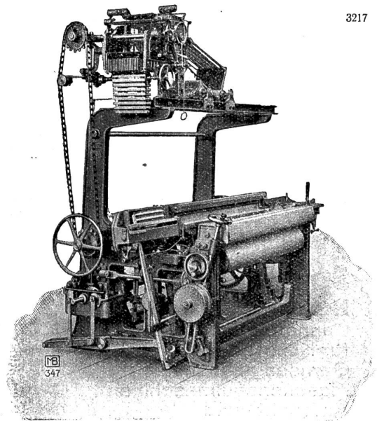
Vierschützig einseitiger Wechselstuhl
